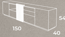
Mueble TV TV Cabinet NA64600 - 400P Lacado Lacquered: 302 / 146 Tirador Handle: 146
