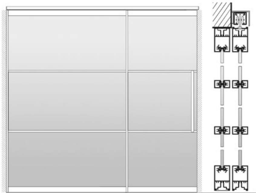
POSIBILIDAD DE FIJO + 1 HOJA CORREDERA
