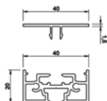
Perfil Base + Tapa
