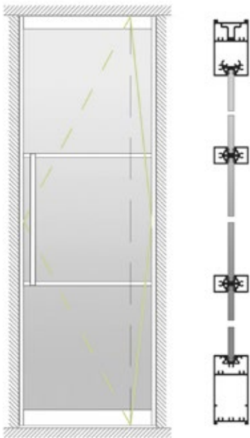
PIVOTANTE 1 HOJA APERTURA D/I
