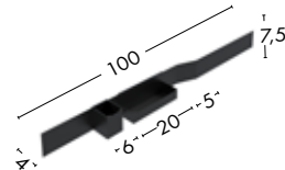
Accesorio metálico
