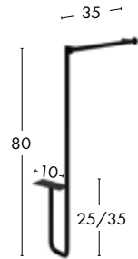
Toallero + pata
